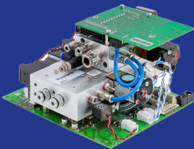
Digitaler Gasmischer
